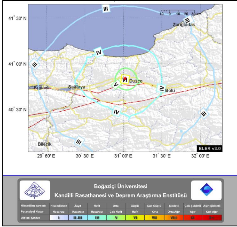
Şekil-5: 17 Kasım 2021 Islahiye-Düzce ( M=5.2 ) Depreminde hemen sonra otomatik olarak üretilen tahmini şiddet dağılım haritasında depremin merkezinde şiddet değeri I_0=VI olarak saptanmıştır
