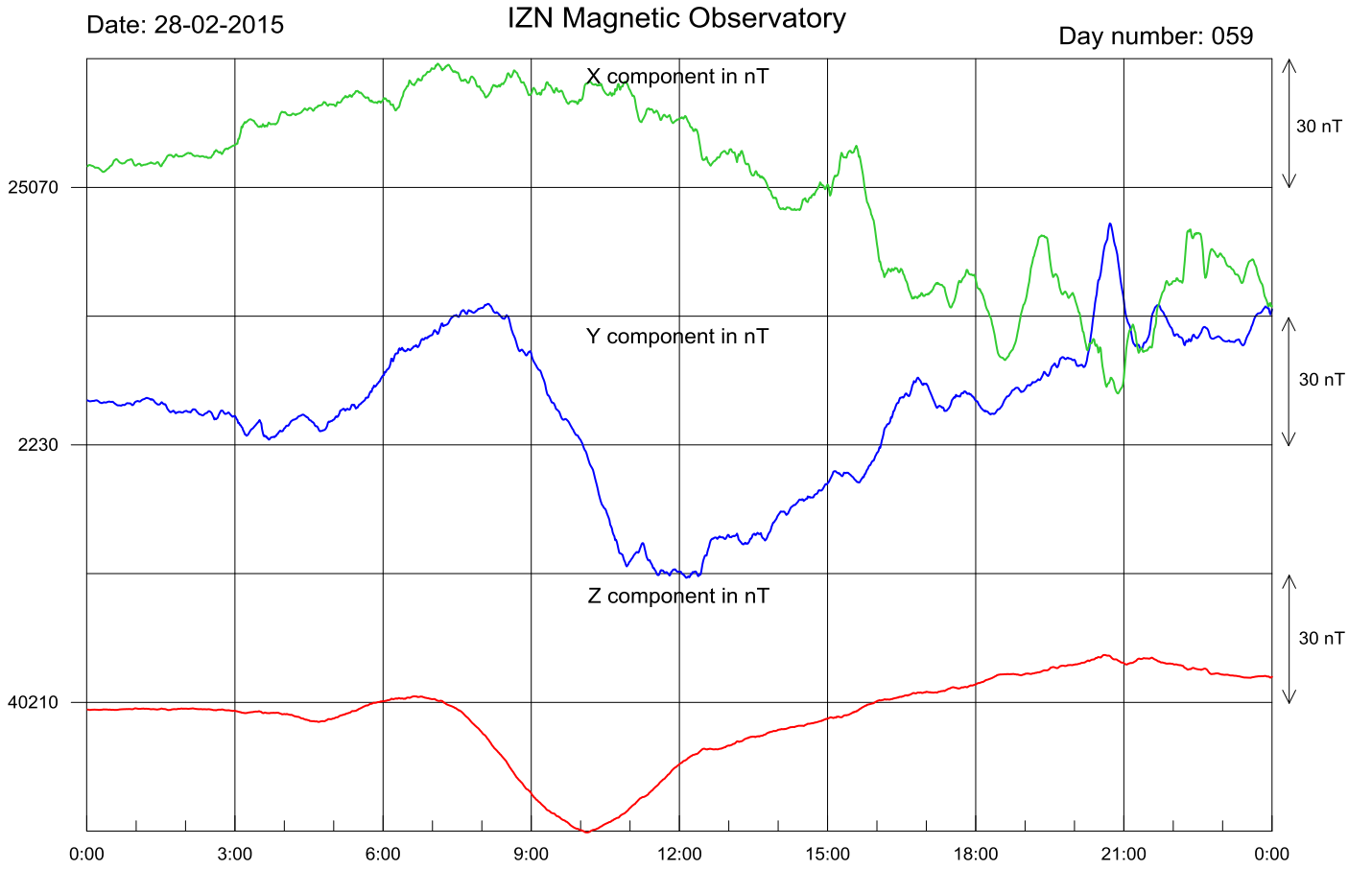
Şekil-1. İznik Manyetik Rasathanesi'nde kaydedilen 2015 Şubat ayı günlük manyetik alan değişimi.
