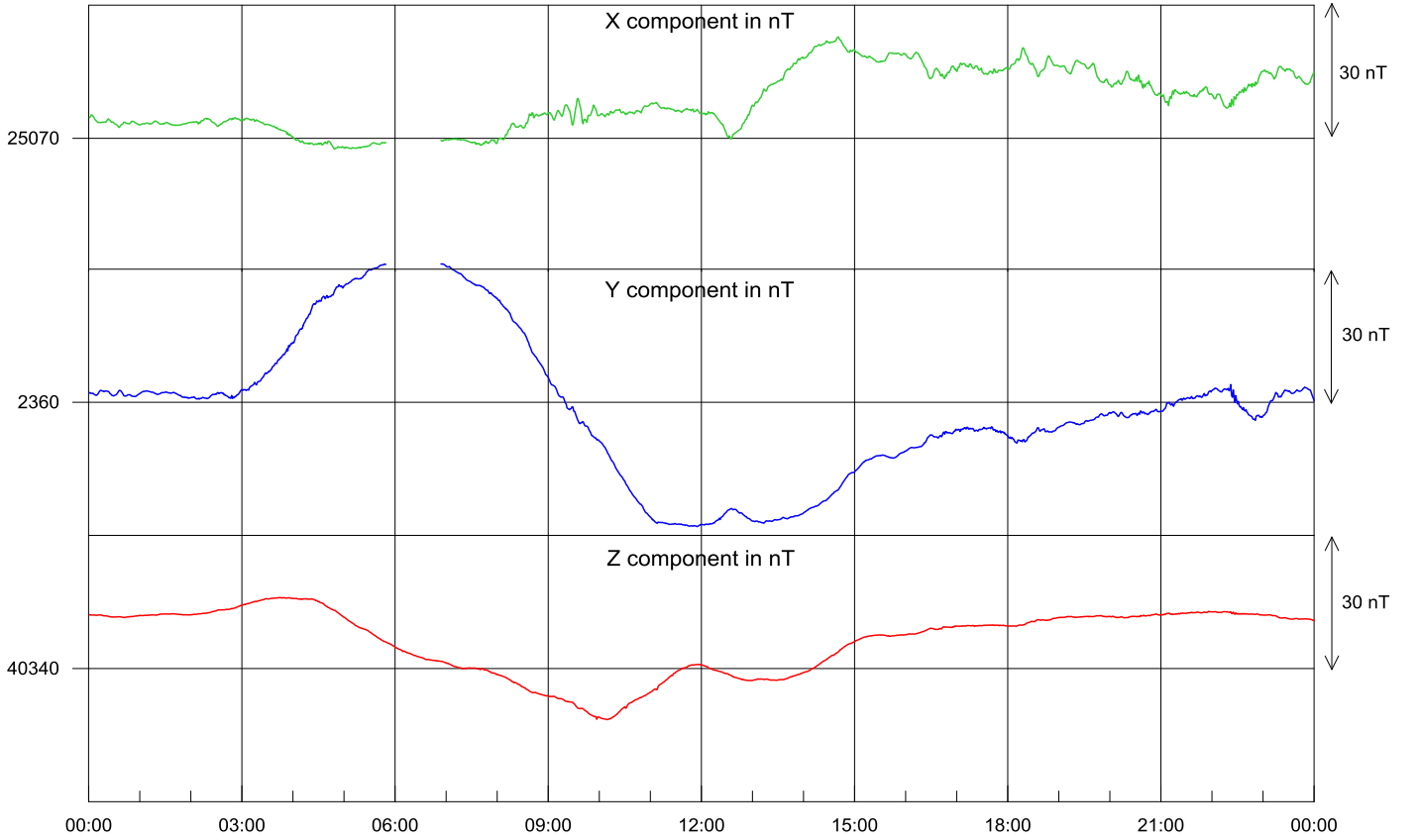
Şekil-1. İznik Manyetik Rasathanesi'nde kaydedilen 2017 Haziran ayı günlük manyetik alan değişimi.
