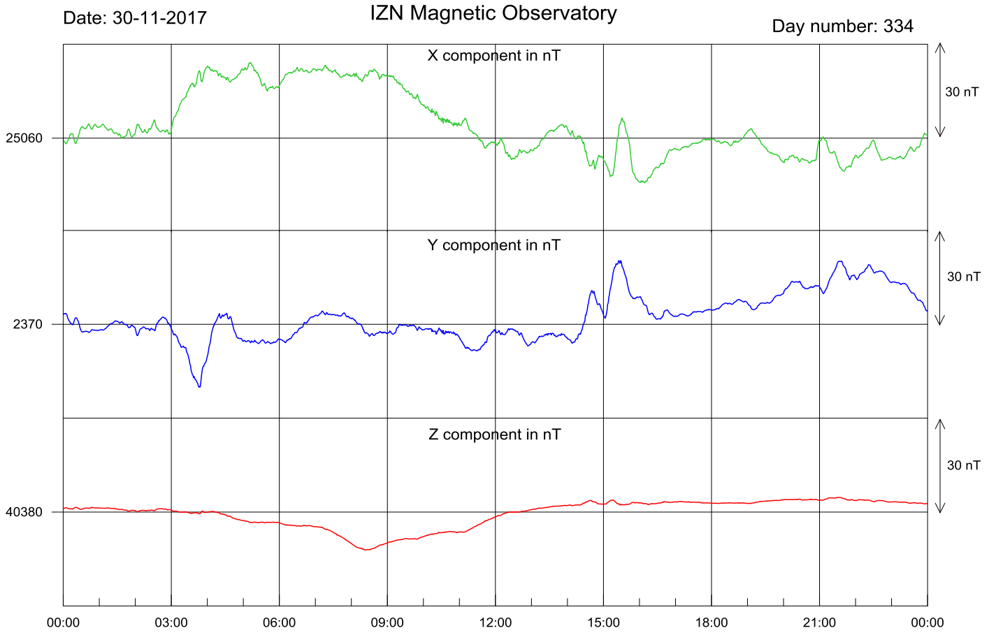
Şekil-1. İznik Manyetik Rasathanesi'nde kaydedilen 2017 Kasım ayı günlük manyetik alan değişimi.
