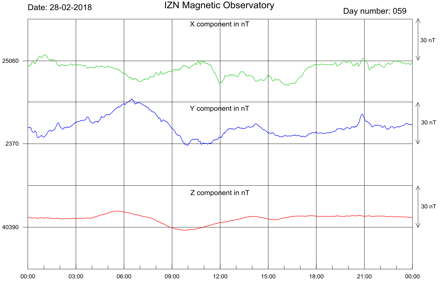
Şekil-1. İznik Manyetik Rasathanesi'nde kaydedilen 2018 Şubat ayı günlük manyetik alan değişimi.
