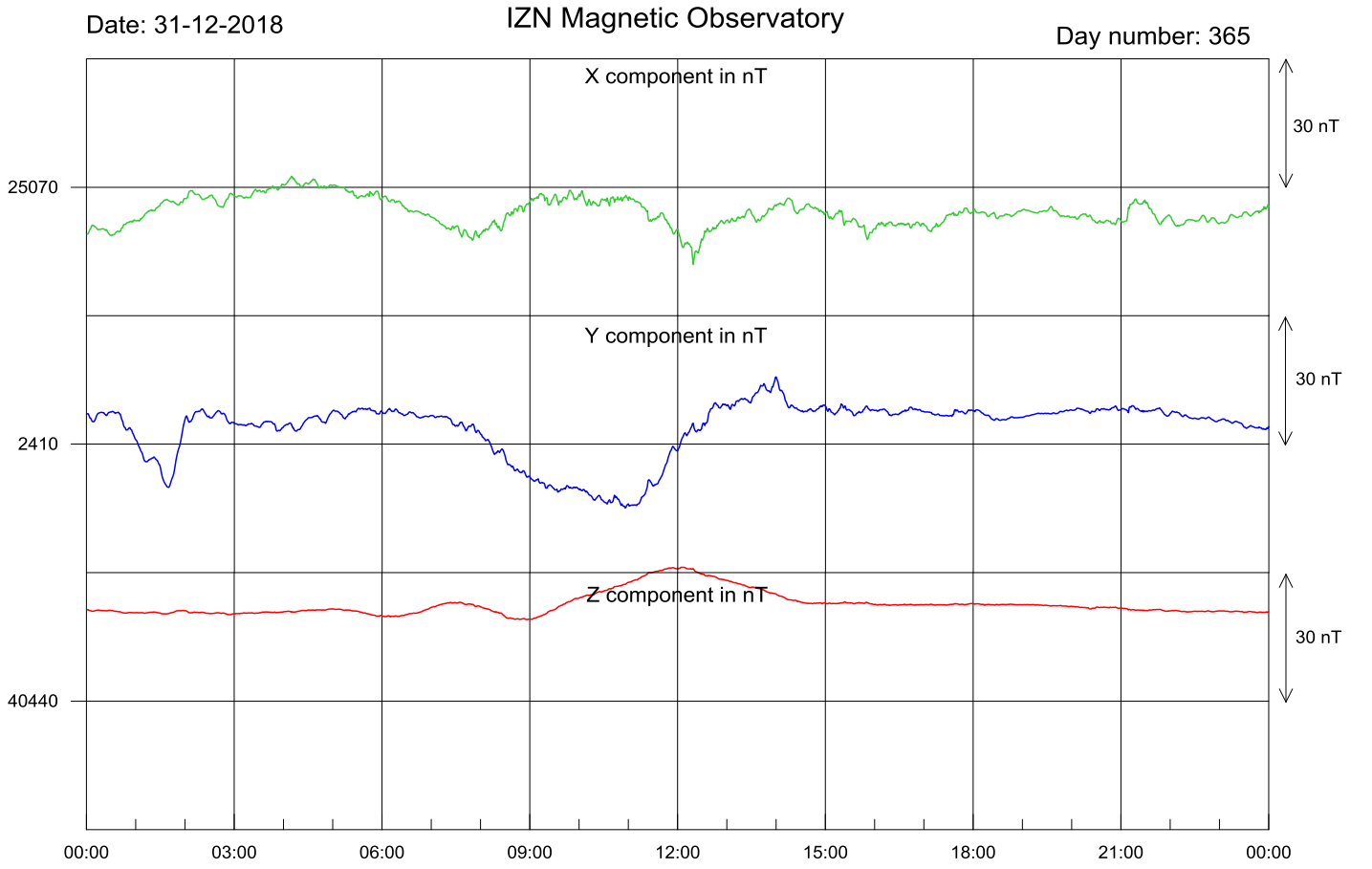
Şekil-1. İznik Manyetik Rasathanesi'nde kaydedilen 2018 Aralık ayı günlük manyetik alan değişimi.
