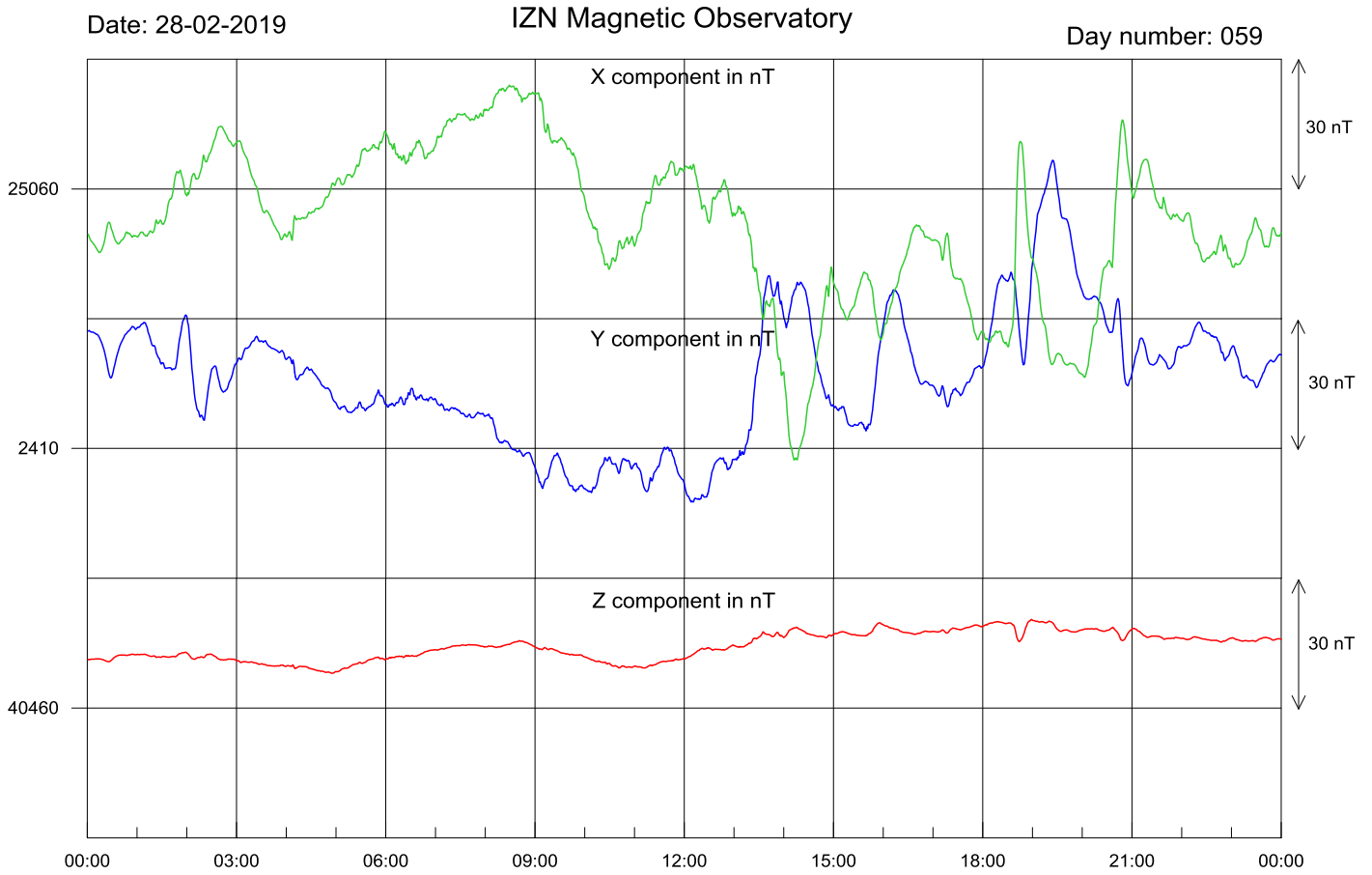
Şekil-1. İznik Manyetik Rasathanesi'nde kaydedilen 2019 Şubat ayı günlük manyetik alan değişimi.
