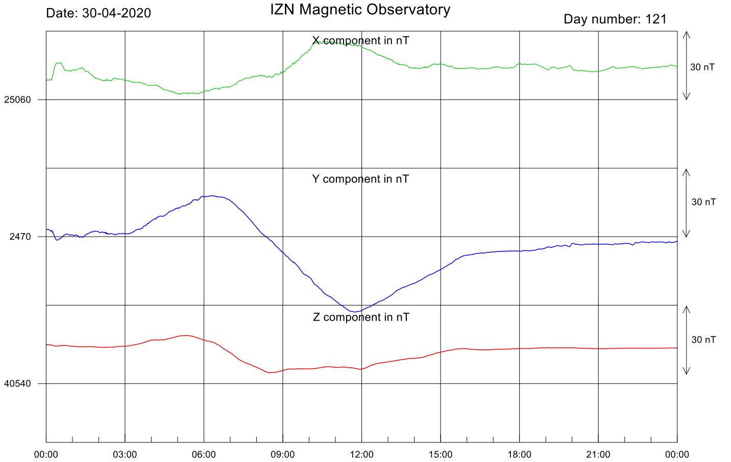
Şekil-1. İznik Manyetik Rasathanesi'nde kaydedilen 2020 Nisan ayı günlük manyetik alan değişimi.
