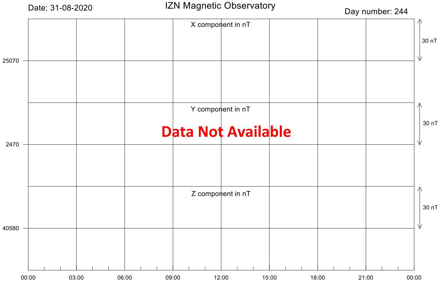
Şekil-1. İznik Manyetik Rasathanesi'nde kaydedilen 2020 Ağustos ayı günlük manyetik alan değişimi.
