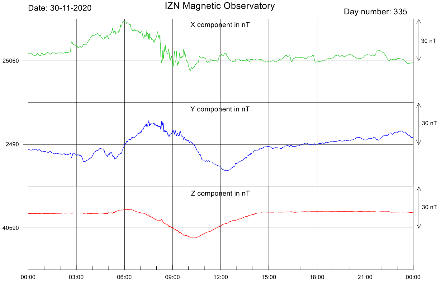
Şekil-1. İznik Manyetik Rasathanesi'nde kaydedilen 2020 Kasım ayı günlük manyetik alan değişimi.
