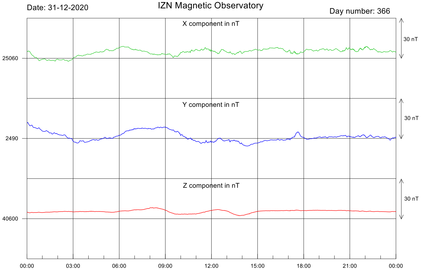
Şekil-1. İznik Manyetik Rasathanesi'nde kaydedilen 2020 Aralık ayı günlük manyetik alan değişimi.
