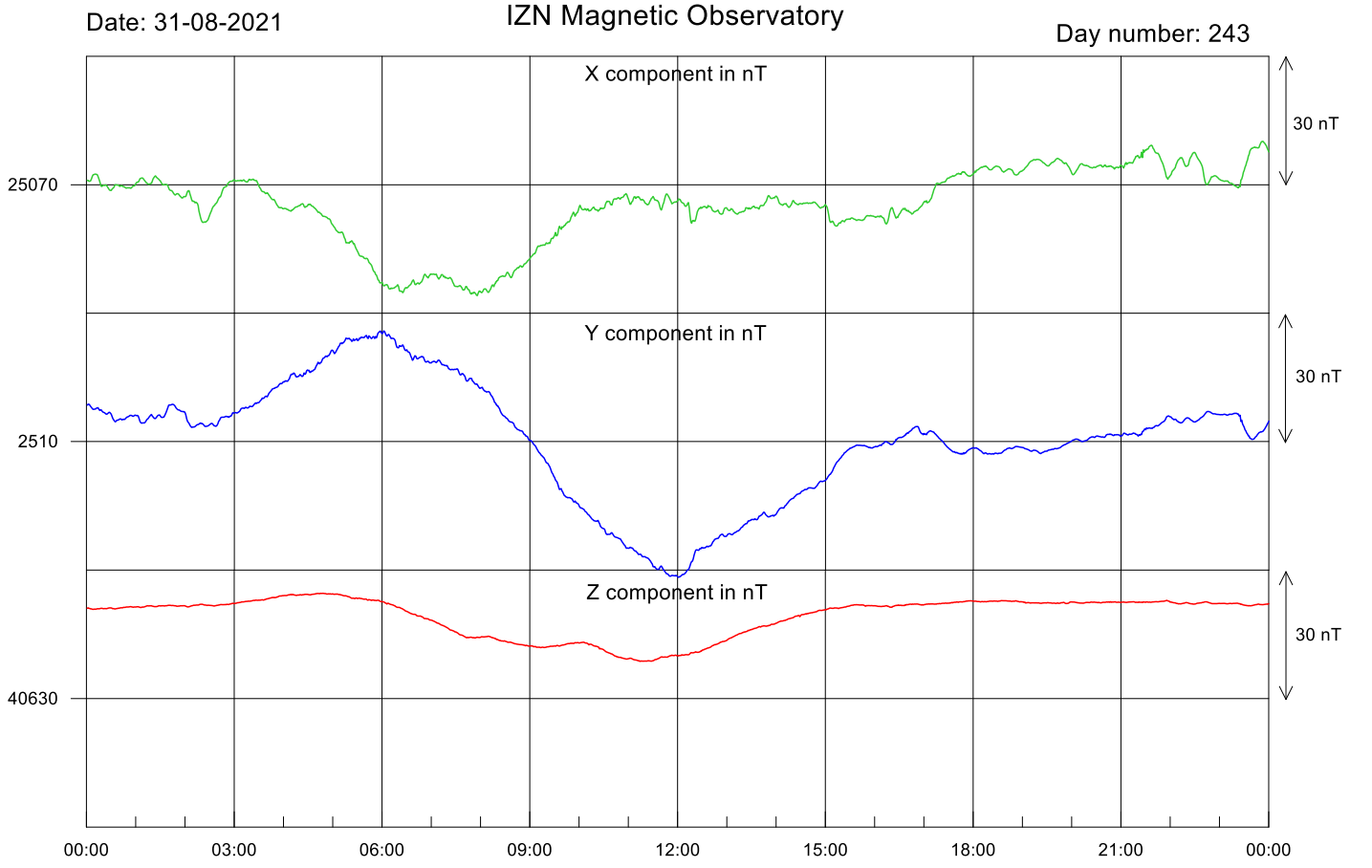
Şekil-1. İznik Manyetik Rasathanesi'nde kaydedilen 2021 Ağustos ayı günlük manyetik alan değişimi.
