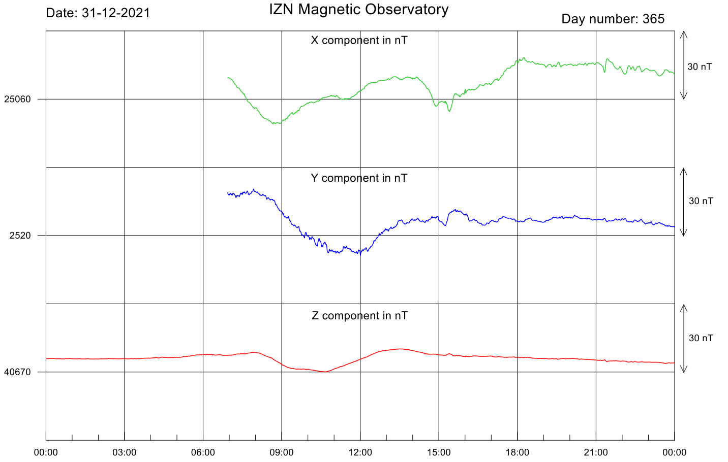
Şekil-1. İznik Manyetik Rasathanesi'nde kaydedilen 2021 Aralık ayı günlük manyetik alan değişimi.
