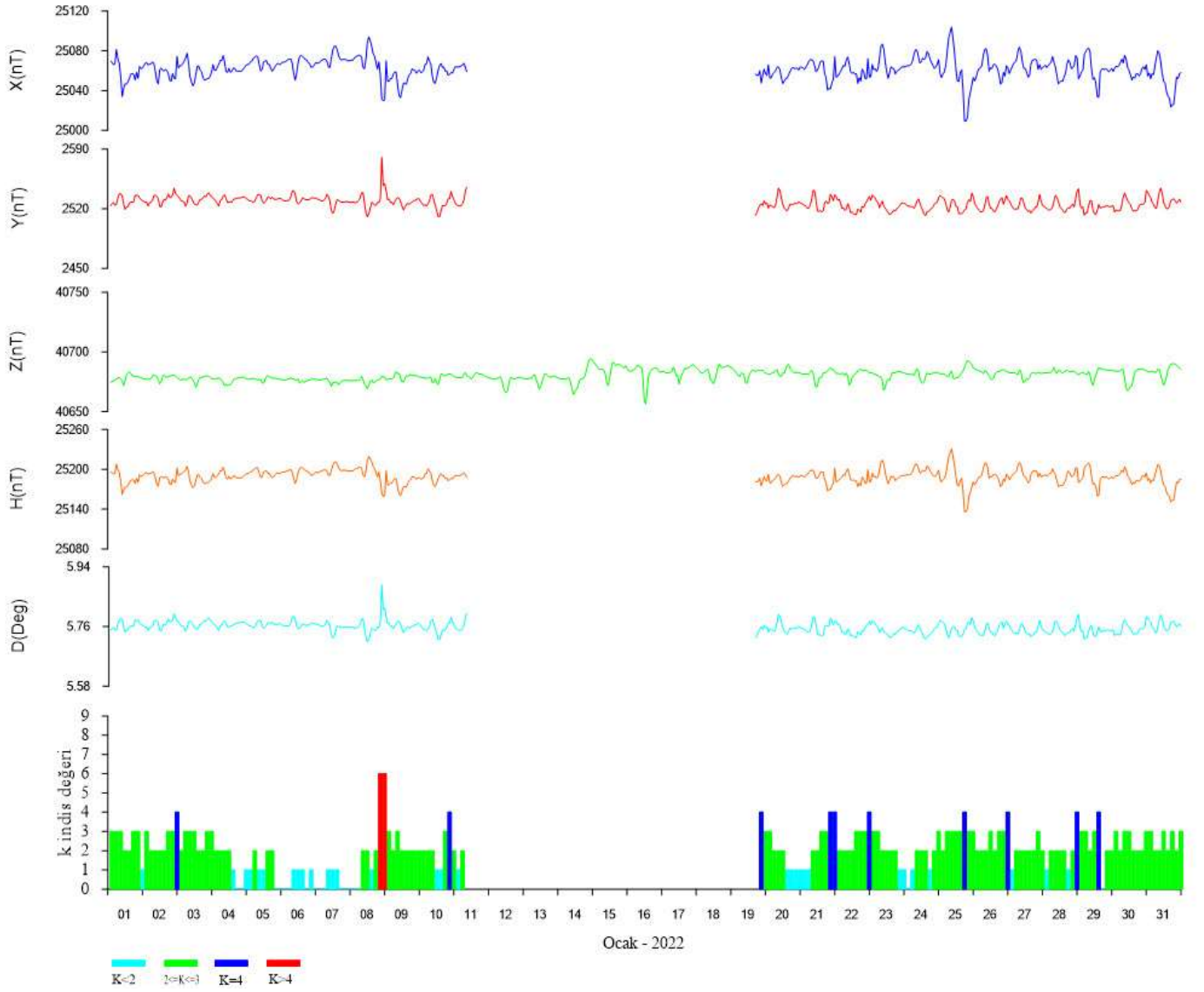
Şekil-2. 2022 Ocak ayı yer manyetik alanın değişimi ve K aktivite değeri.
