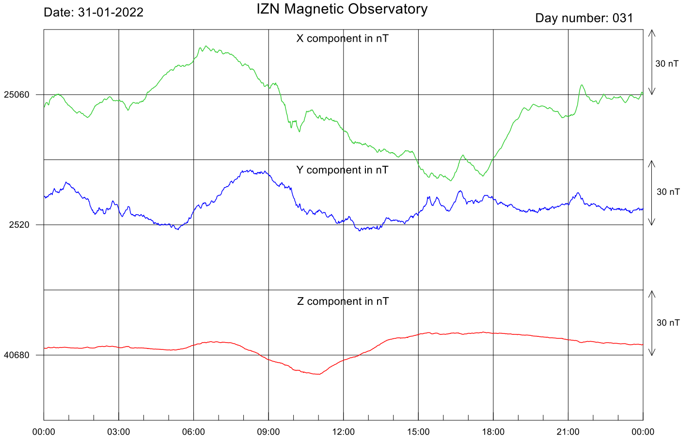
Şekil-1. İznik Manyetik Rasathanesi'nde kaydedilen 2022 Ocak ayı günlük manyetik alan değişimi.
