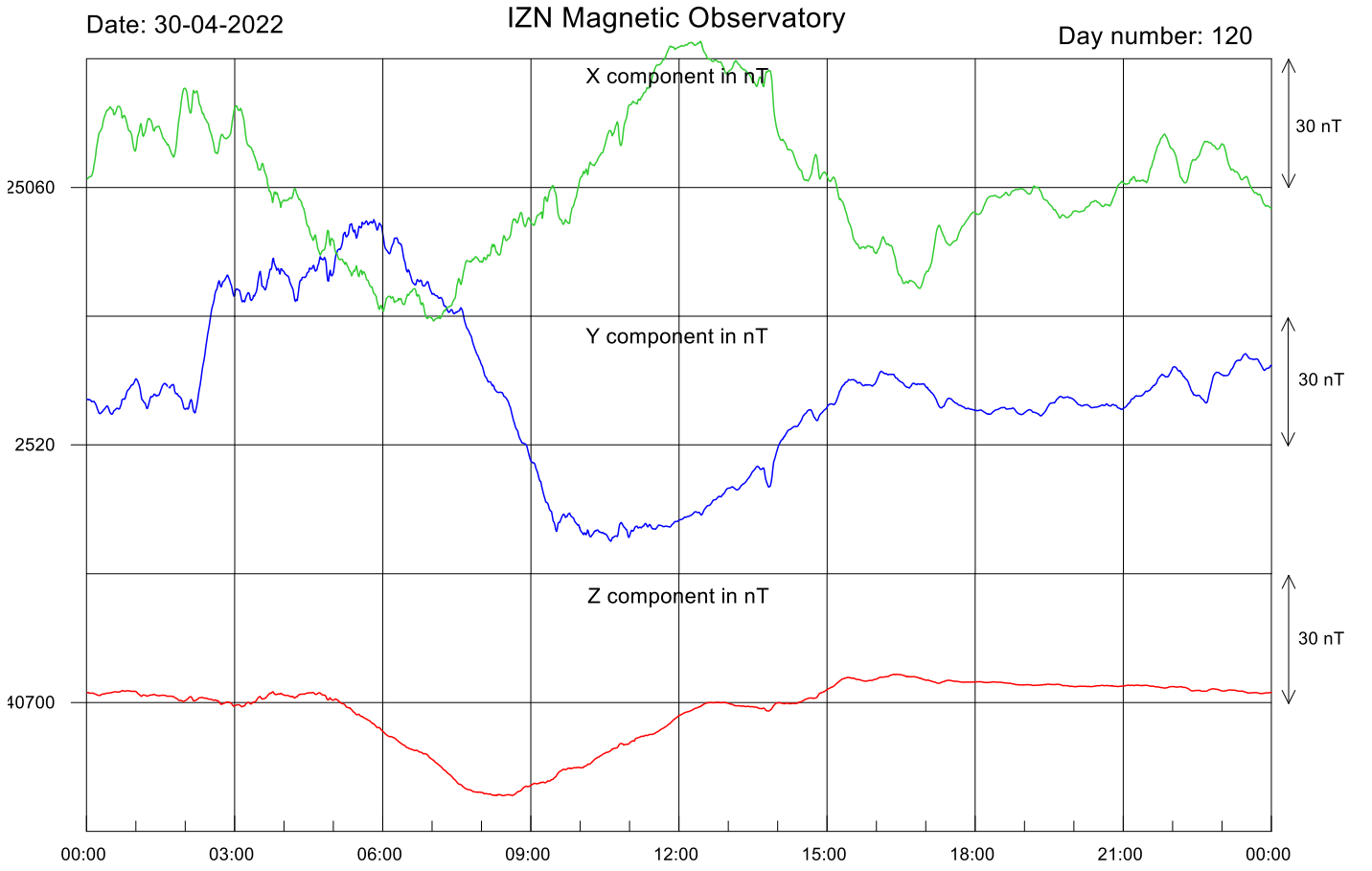
Şekil-1. İznik Manyetik Rasathanesi'nde kaydedilen 2022 Nisan ayı günlük manyetik alan değişimi.
