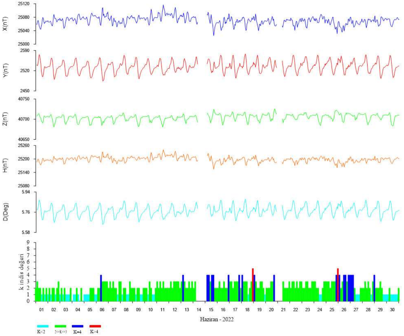
Şekil-2. 2022 Haziran ayı yer manyetik alanın değişimi ve K aktivite değeri.
