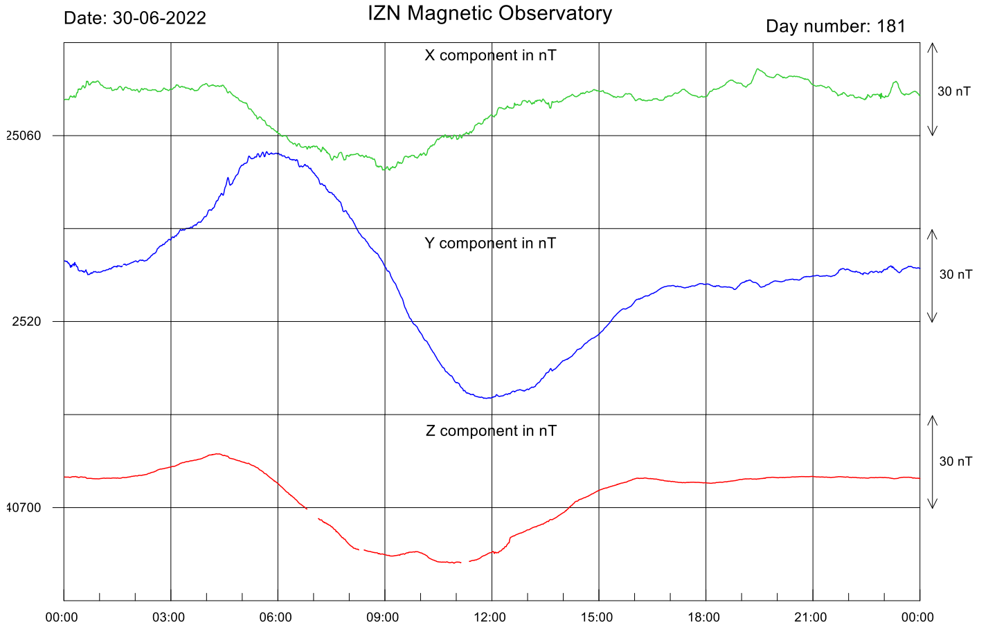
Şekil-1. İznik Manyetik Rasathanesi'nde kaydedilen 2022 Haziran ayı günlük manyetik alan değişimi.
