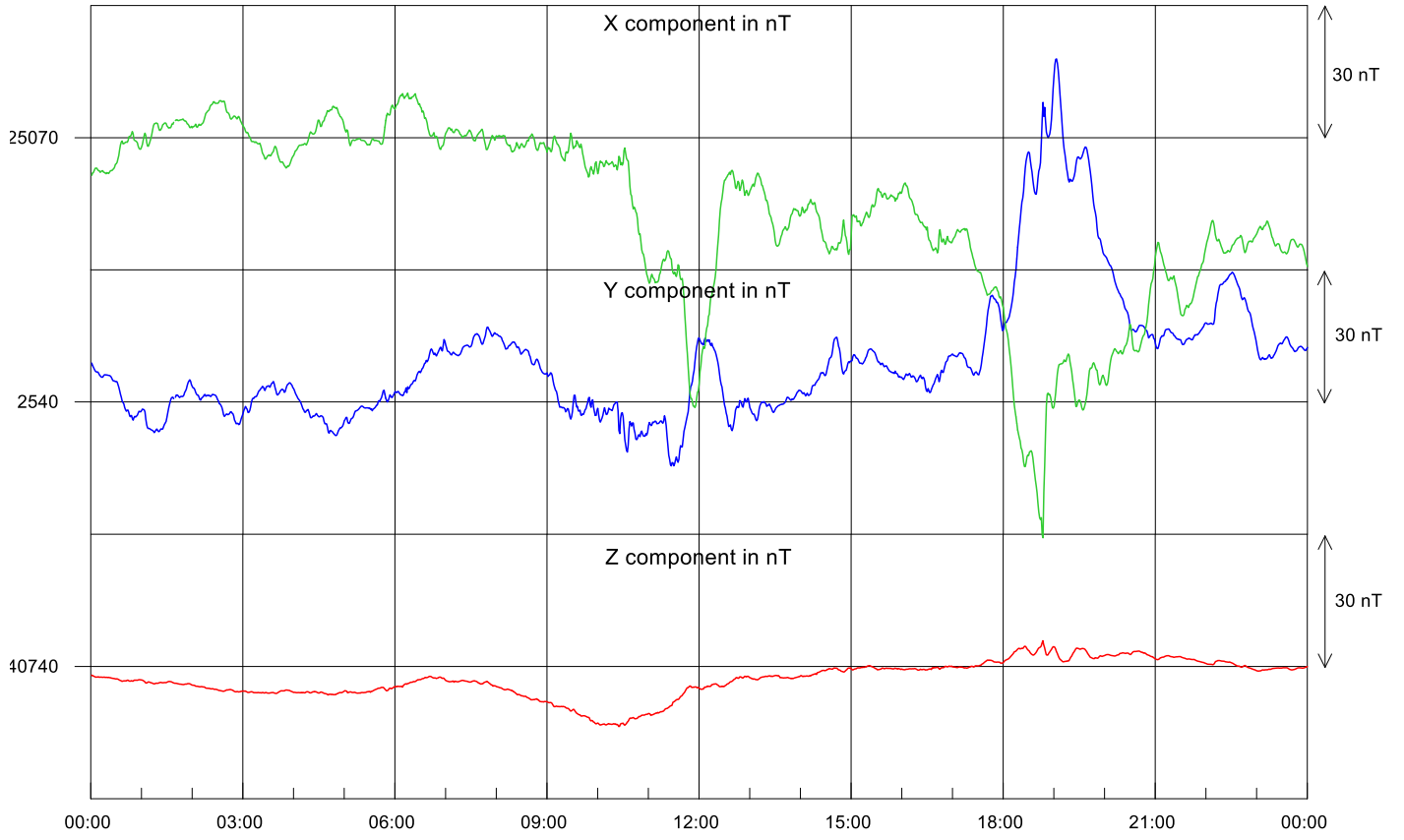
Şekil-1. İznik Manyetik Rasathanesi'nde kaydedilen 2022 Kasım ayı günlük manyetik alan değişimi.
