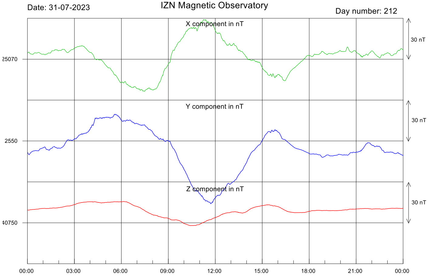
Şekil-1. İznik Manyetik Rasathanesi'nde kaydedilen 2023 Temmuz ayı günlük manyetik alan değişimi.
