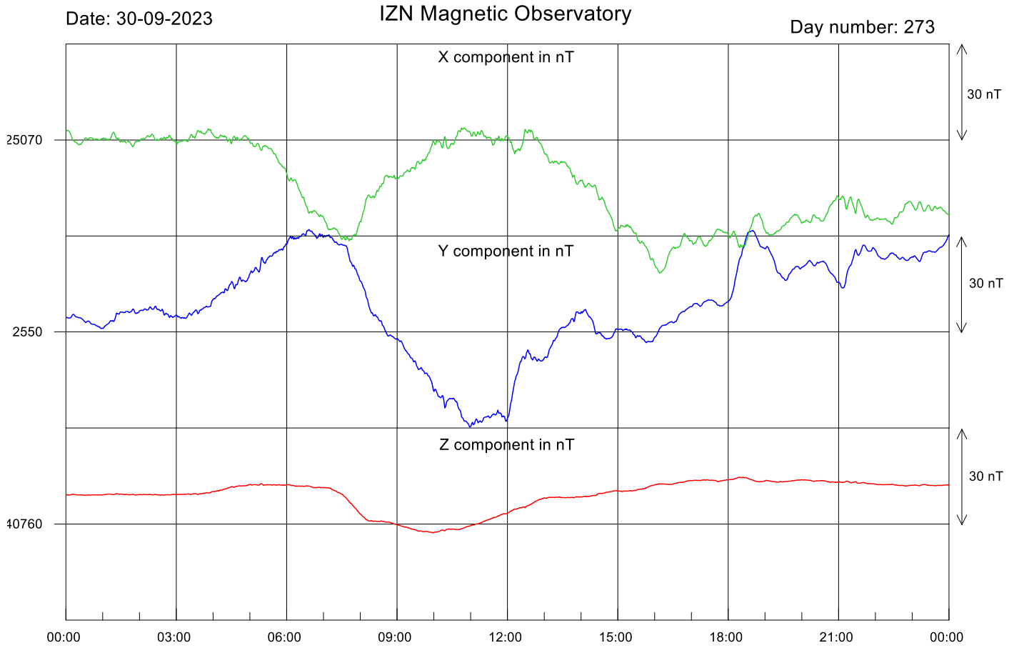
Şekil-1. İznik Manyetik Rasathanesi'nde kaydedilen 2023 Eylül ayı günlük manyetik alan değişimi.
