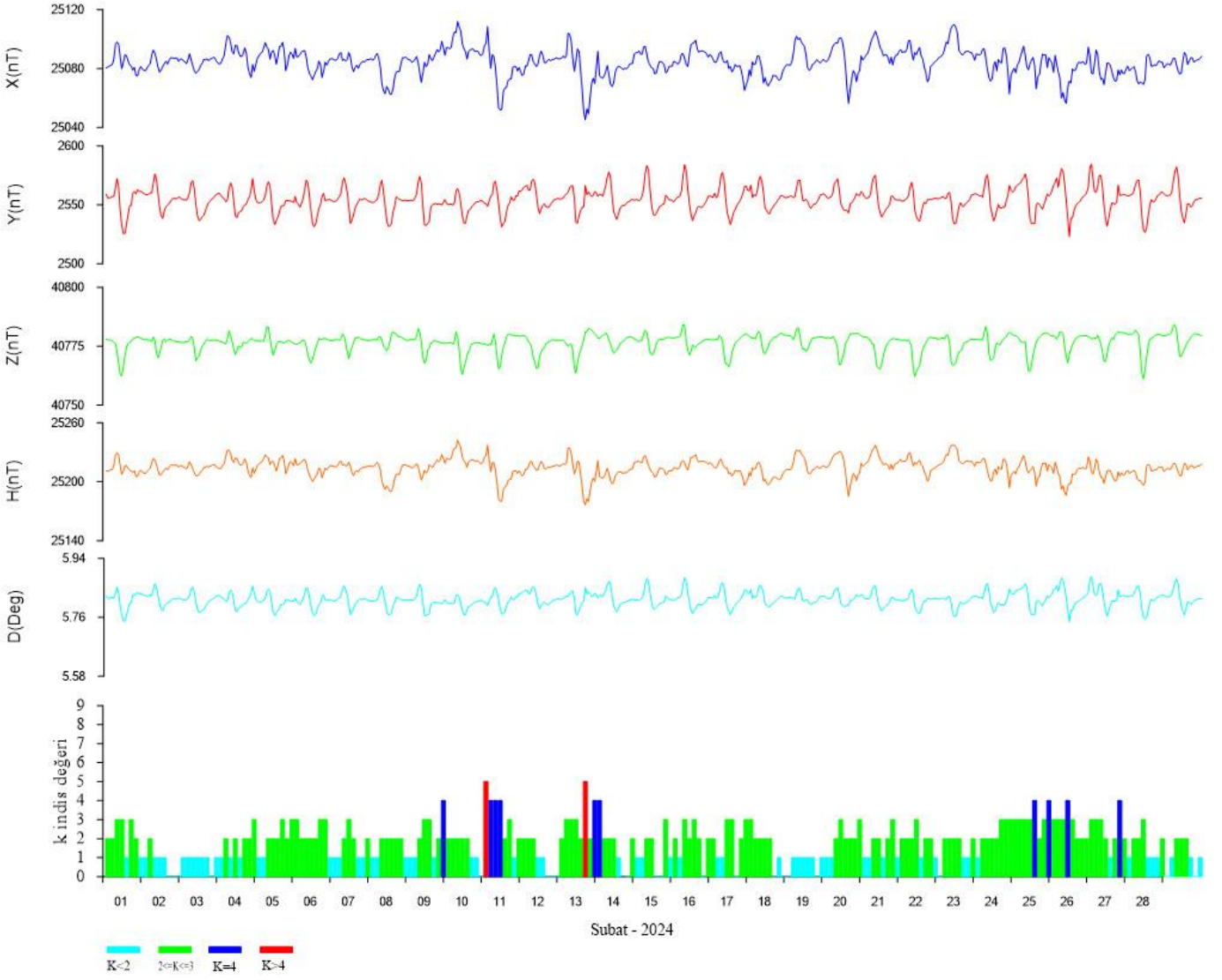
Şekil-2. 2024 Şubat ayı yer manyetik alanın değişimi ve K aktivite değeri.
