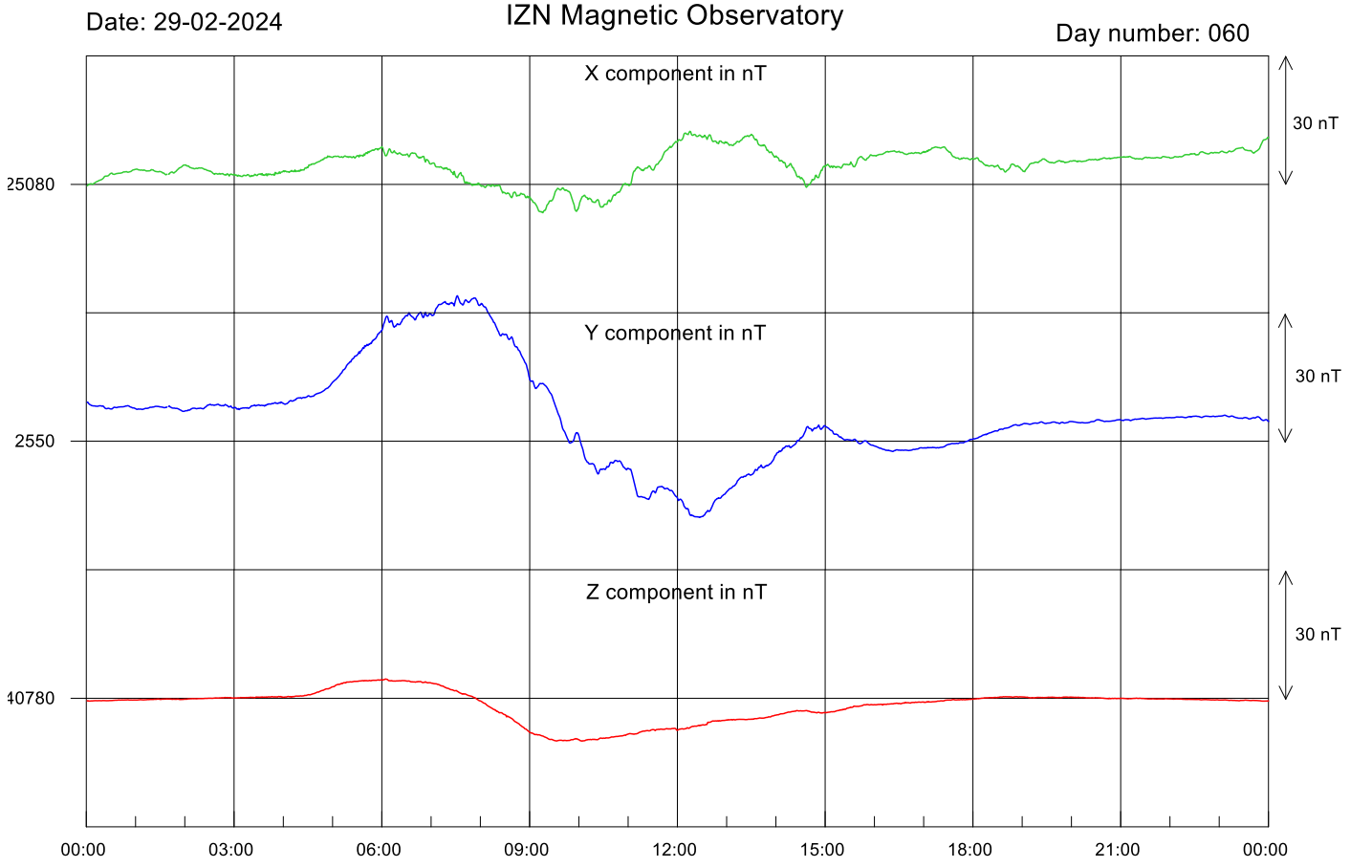
Şekil-1. İznik Manyetik Rasathanesi'nde kaydedilen 2024 Şubat ayı günlük manyetik alan değişimi.
